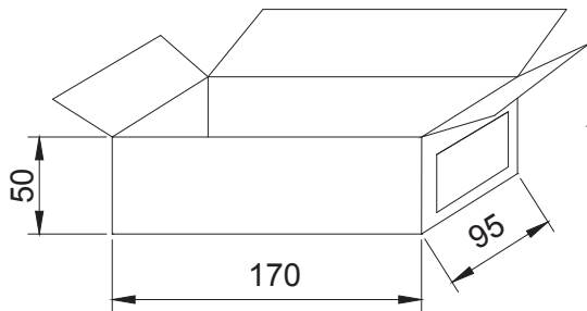
Inner box (1bag max/box)
