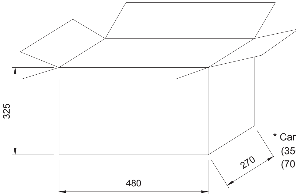
Inner box (1bag max/box)
